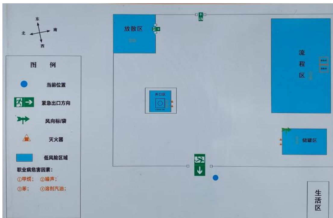
图 2.5-1 采气工程井场平面布局现状图
