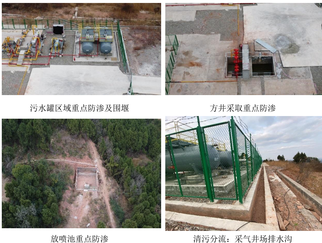
图 6.2-1 部分地下水防治措施现状图
